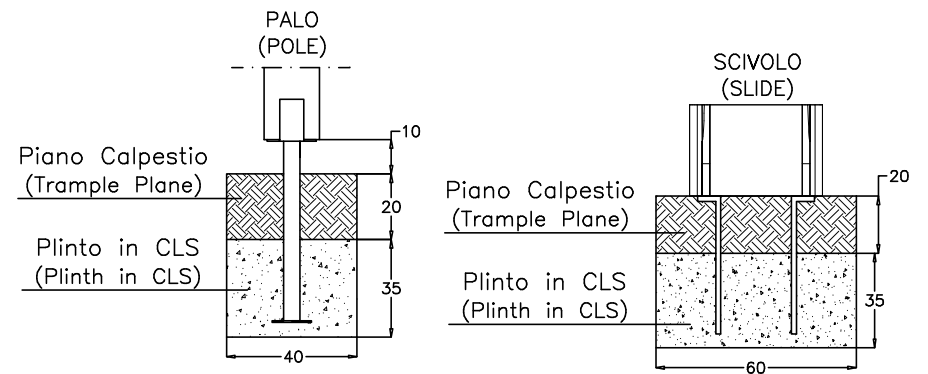
PARTICOLARI ANCORAGGIO (ANCHORAGE DETAIL)
