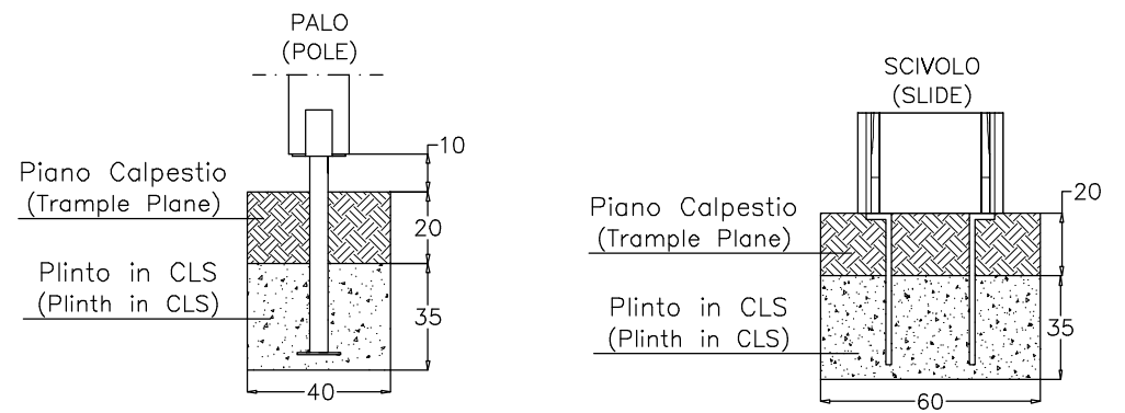
PARTICOLARI ANCORAGGIO (ANCHORAGE DETAIL)
