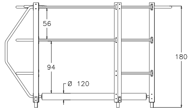
LATERALE (LATERAL)
