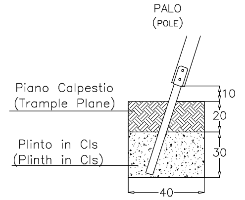
PARTICOLARI ANCORAGGIO (ANCHORAGE DETAIL)
