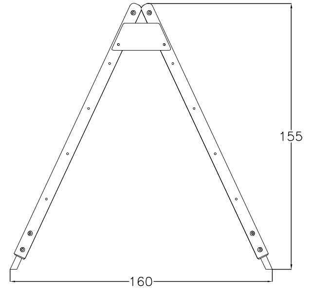
LATERALE (LATERAL)
