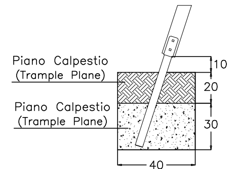
PARTICOLARI ANCORAGGIO (ANCHORAGE DETAIL)
